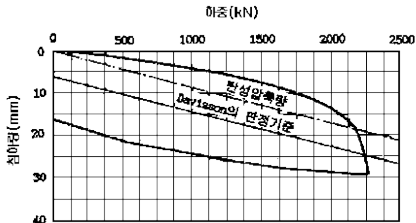
[그림 14] 항타종료후 14일에 실시된 정재하시험결과 (after Preim등, 1989)
