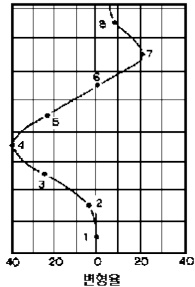
b) 말뚝관입으로 인한 변형율
