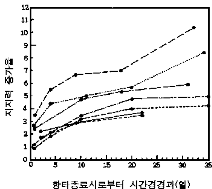
[그림 17] 점성토지반에서의 시간경과에 따른 말뚝지지력 증가율 - 항타종료시 대비(after Svinkin 등, 1994)
